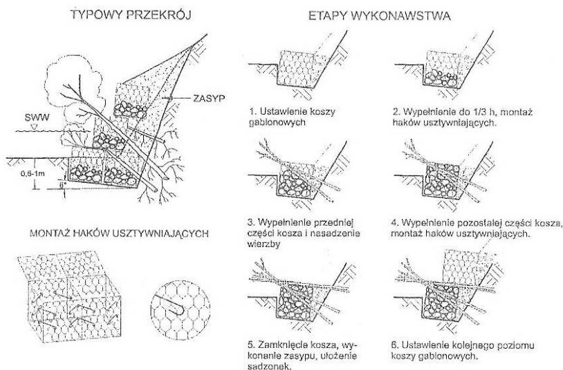
Rys. 9. Kosze gabionowe z nasadzeniami (Bednarczyk, Duszyński 2008: 200)
