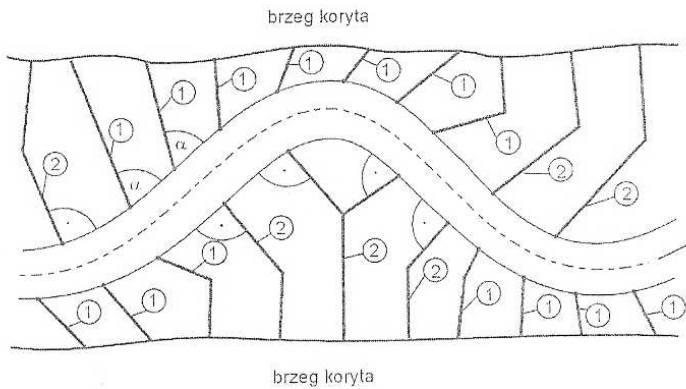
Rys.3. Usytuowanie ostróg podprądowych (1) i prądowych (2) na łukach trasy regulacyjnej rzeki (Bednarczyk, Duszyński 2008: 159)
